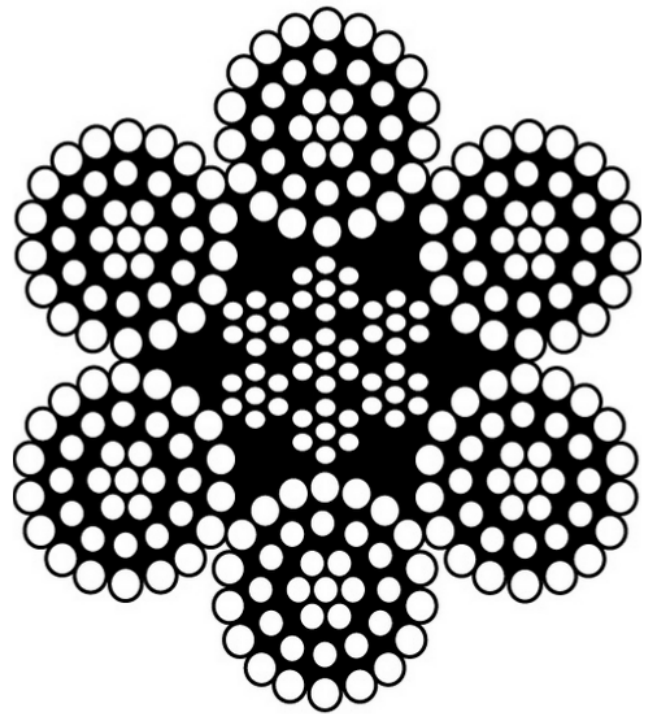
6 X 37
