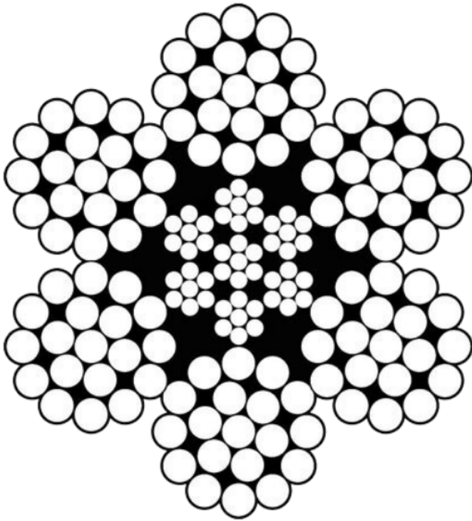
6 X 19
